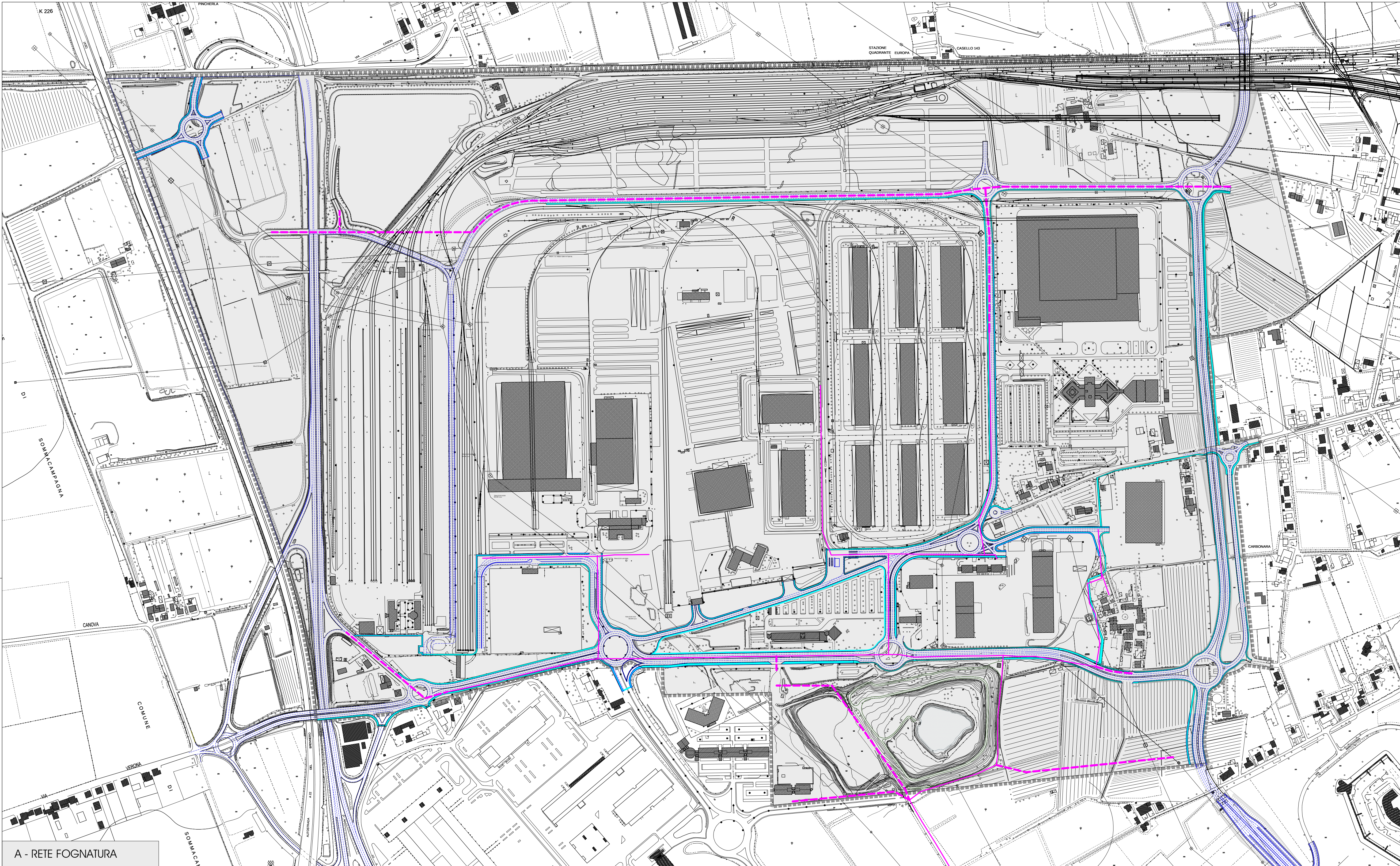
A - RETE FOGNATURA
